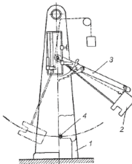
1 – стойки; 2 – маятник; 3 – подъемная рама; 4 – образец
