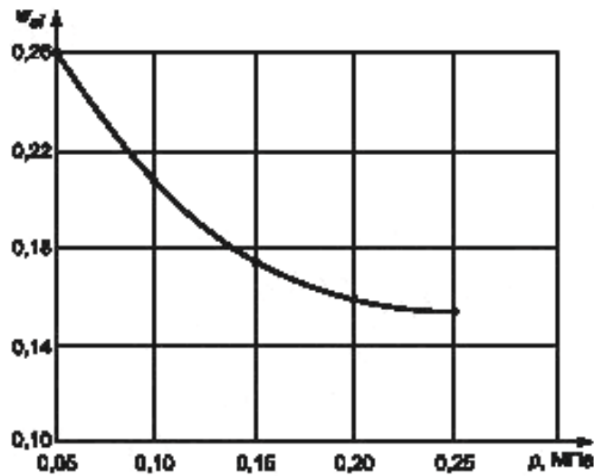
б) График зависимости начальной просадочной влажности w_{s1} от давления p
