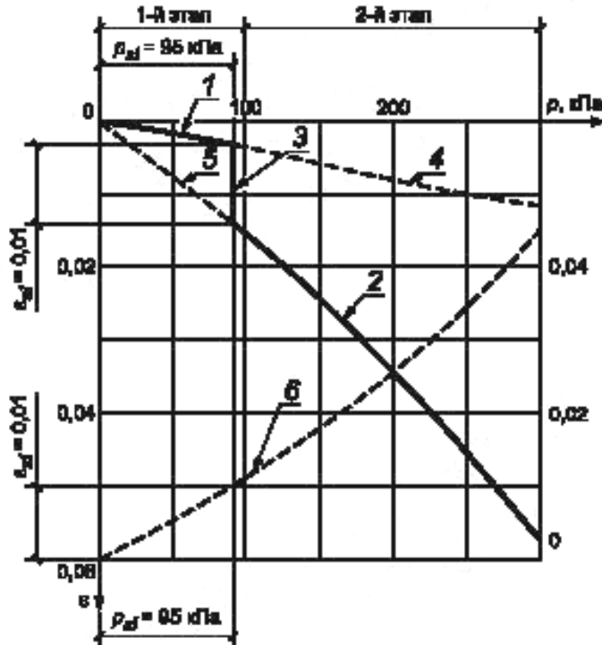
Рисунок В.1 — График испытания просадочного грунта ускоренным методом по «комбинированной схеме»
