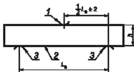
1 — опора для приложения нагрузки (нажимная); 2 — поверхность образца, работающая на растяжение; 3 — опоры, поддерживающие образец
