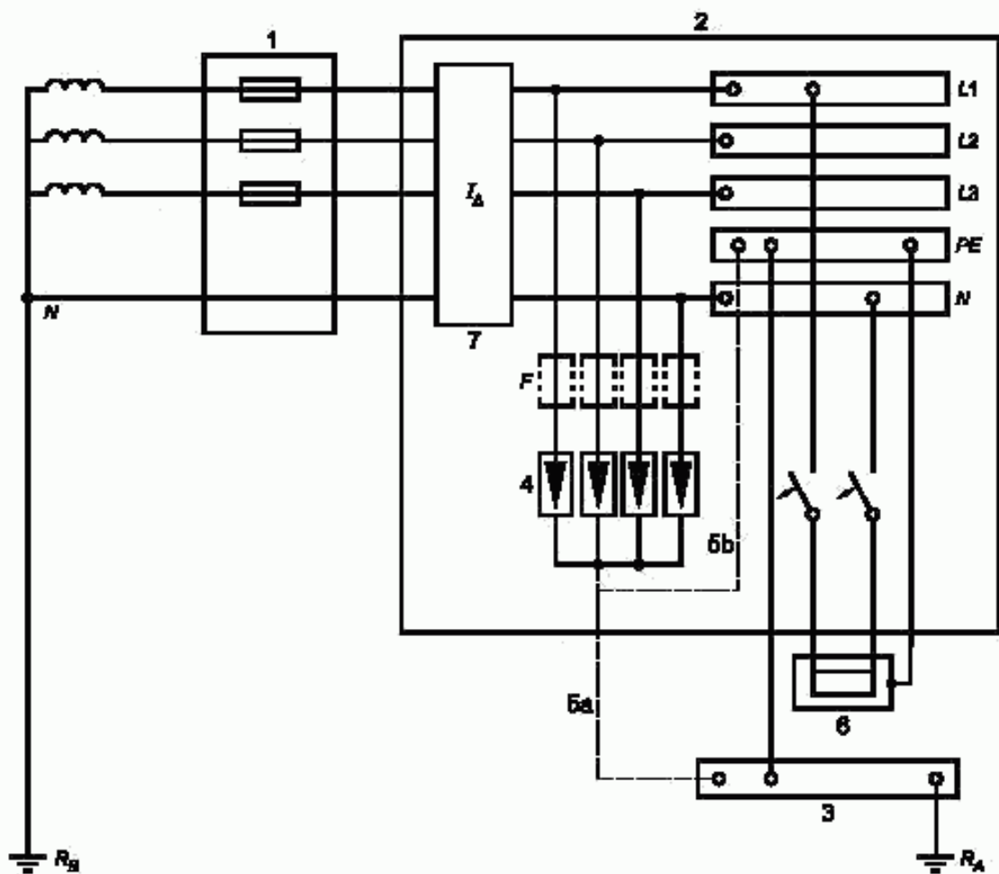
1 — ввод распределительной сети; 2 — распределительный щит; 3 — главный заземляющий зажим (шина); 4 — УЗИП; 5а, 5б — заземление УЗИП; 6 — защищаемое оборудование; 7 — УДТ; F — защитное устройство, указанное изготовителем (предохранитель, автоматический выключатель, УДП); R_A — заземляющий электрод (сопротивление); R_B — заземляющий электрод (сопротивление) системы питания
