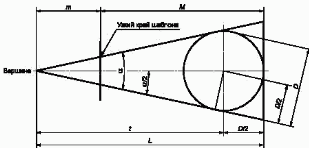
Рисунок Д.3 — Геометрические соотношения для V-образного шаблона
