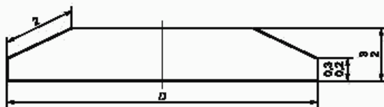
Рисунок Д.2 — Калибровочный диск
