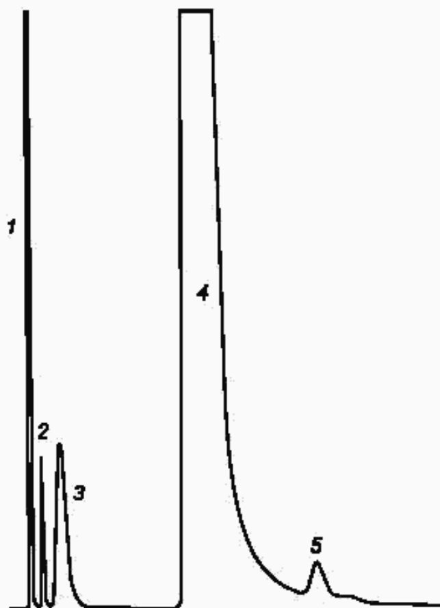
1 — диэтиловый эфир; 2 — н-октан — «внутренний эталон»; 3 — уксусный альдегид; 4 — этиловый спирт; 5 — кротоновый альдегид
