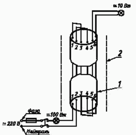
1 — образец кабеля; 2 — трехсторонняя металлическая камера
