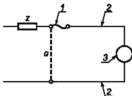
1 — предохранитель; 2 — испытуемый проводник; 3 — защитное устройство двигателя Комплектуемые изделия Z — импеданс для регулирования тока до ожидаемой силы тока в таблице 17.101.1. G — временное присоединение для регулирования тока до ожидаемой силы тока
