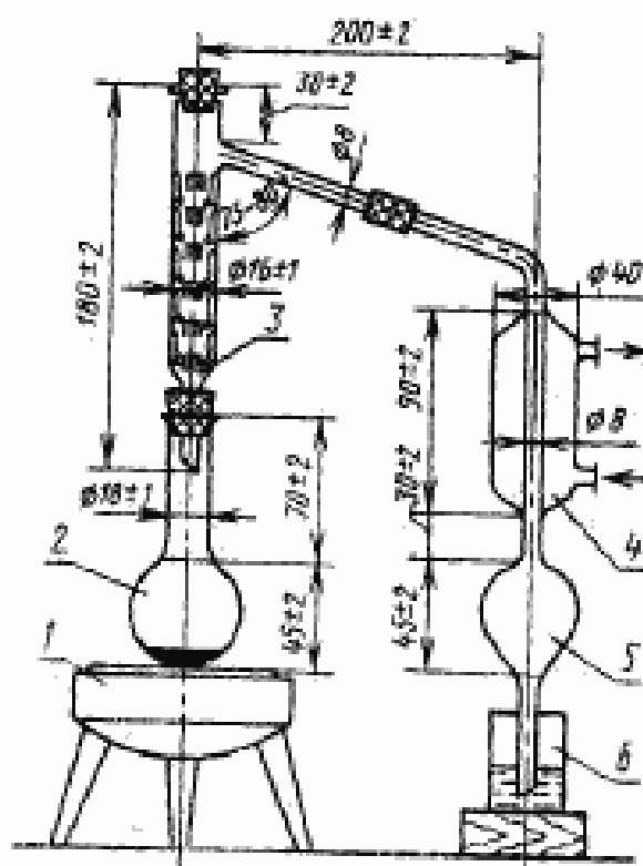
Прибор для дистилляции
