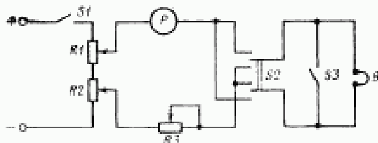
R1-R3 — магазин сопротивлений класса точности 0,5; B — гальванометр; S1, S3 — выключатели; S2 — переключатель направления тока; P — микроамперметр или миллиамперметр постоянного тока класса точности 0,5
