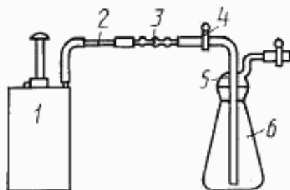
1 — газоанализатор УГ-2; 2 — индикаторная трубочка; 3 — фильтрующий патрон; 4 — зажимы пружинящие; 5 — пробка-насадка Дрекселя; 6 — колба коническая
