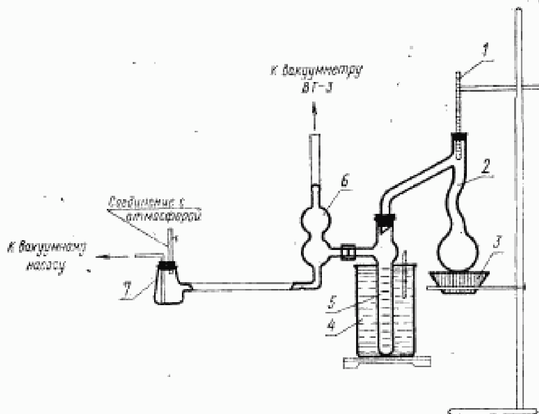
Схема аппарата для перегонки парафина под вакуумом
