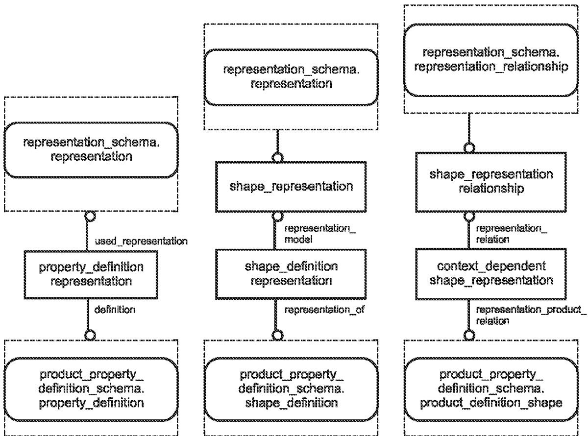
Рисунок F.4 — product_property_representation_schema — EXPRESS-G диаграмма 1 из 1
