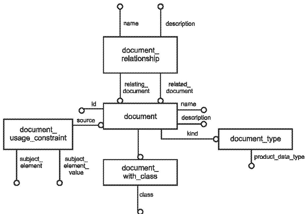
Рисунок F.6 — document_schema — EXPRESS-G диаграмма 1 из 1
