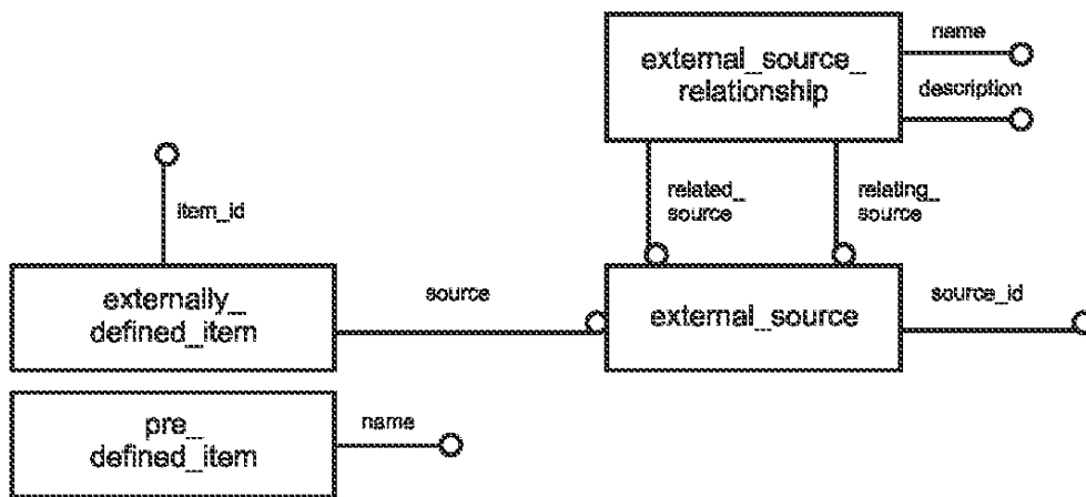
Рисунок F.16 — external_reference_schema — EXPRESS-G диаграмма 1 из 1
