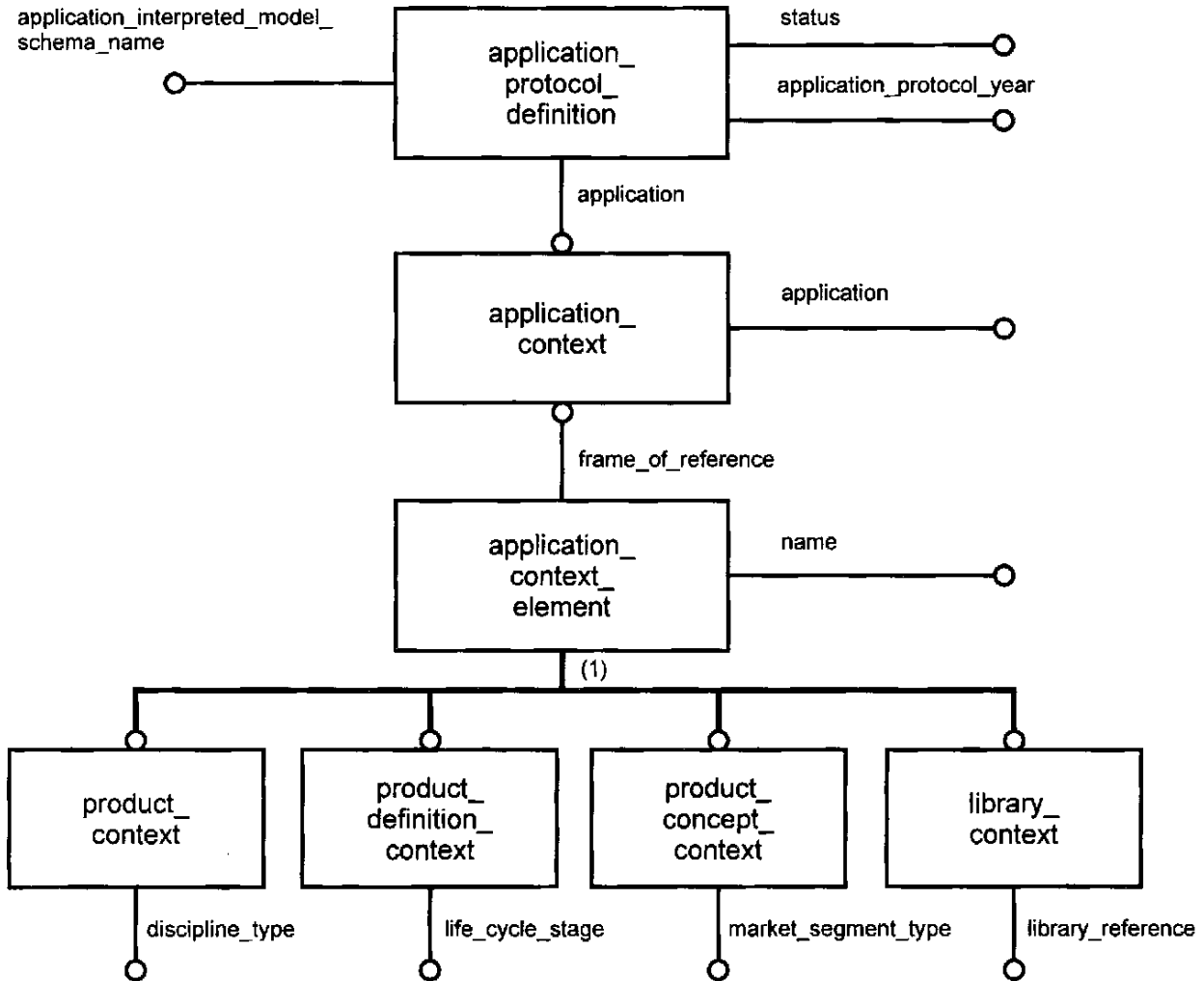
Рисунок F.1 — application_context_schema — EXPRESS-G диаграмма 1 из 1
