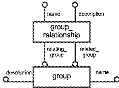
Рисунок F.14 — group_schema — EXPRESS-G диаграмма 1 из 1
