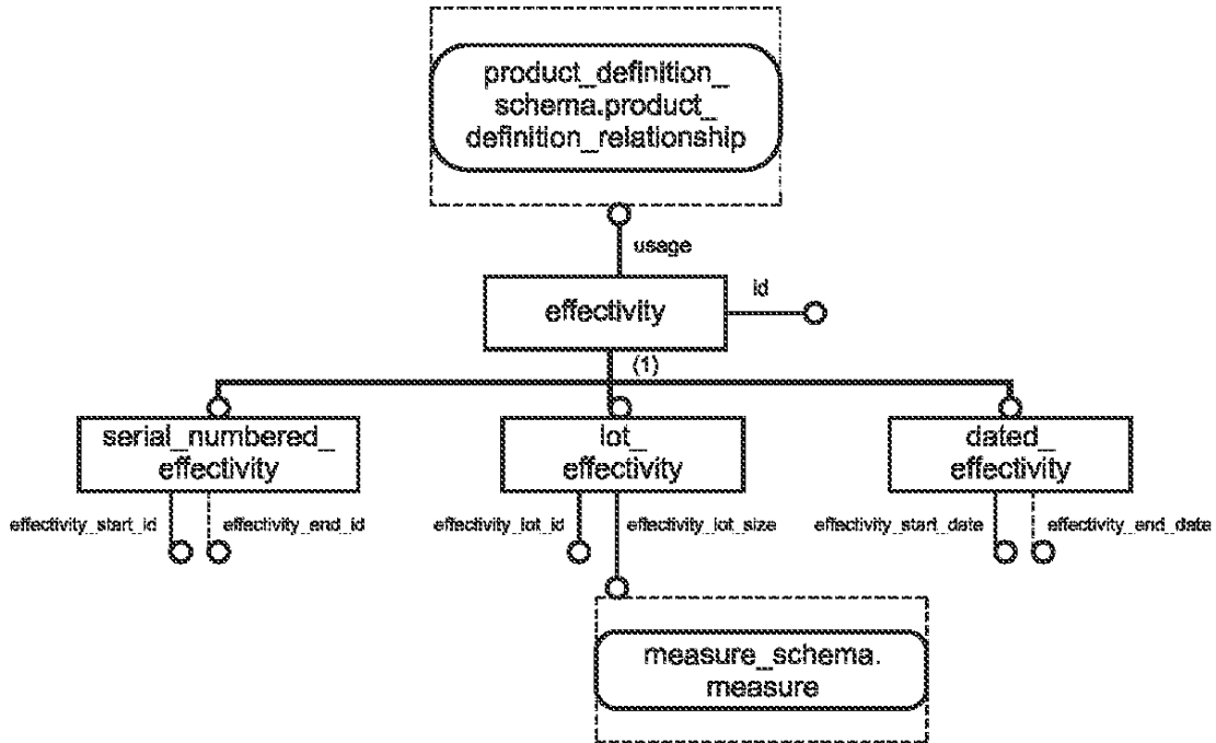
Рисунок F.15 — effectivity_schema — EXPRESS-G диаграмма 1 из 1
