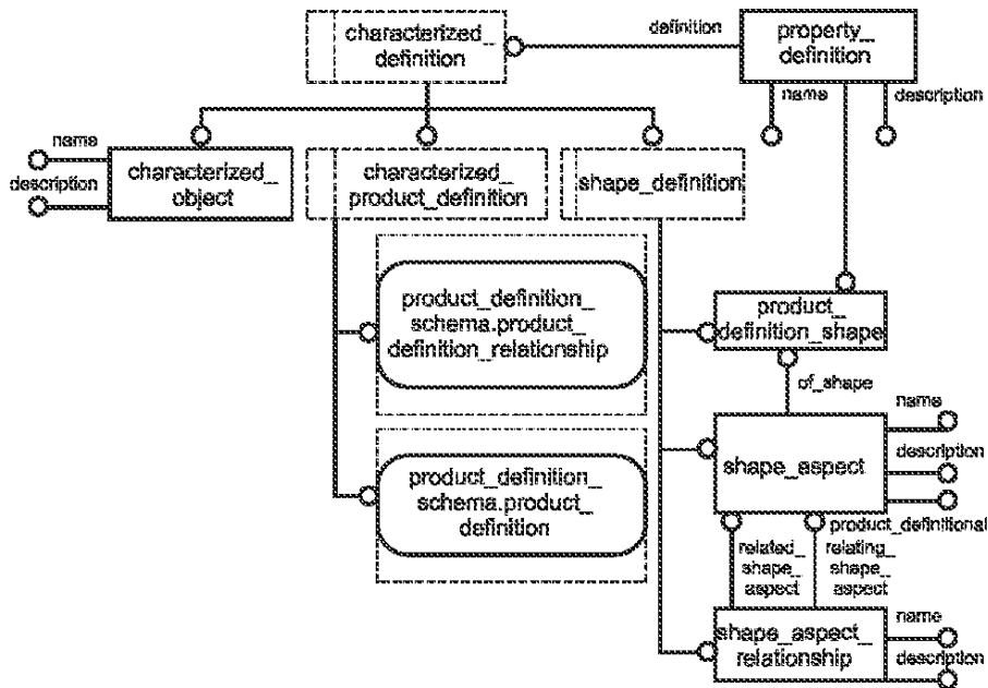
Рисунок F.3 — product_property_definition_schema — EXPRESS-G диаграмма 1 из 1
