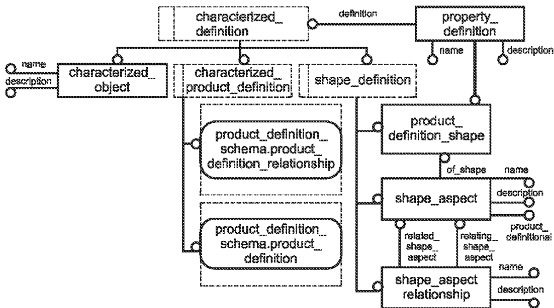
Рисунок F.20 — measure_schema — EXPRESS-G диаграмма 3 из 3
