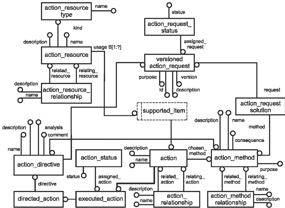
Рисунок F.7 — action_schema — EXPRESS-G диаграмма 1 из 1
