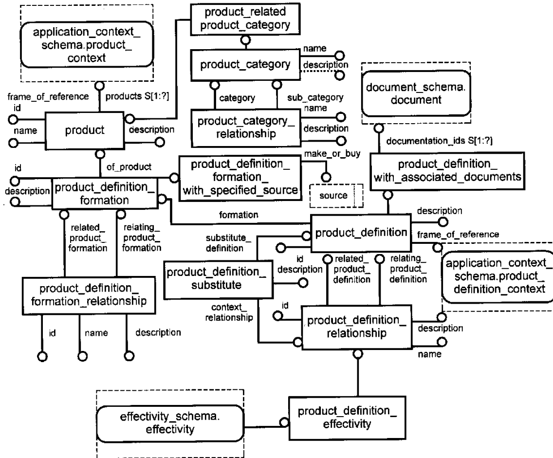
Рисунок F.2 — product_definition_schema — EXPRESS-G диаграмма 1 из 1
