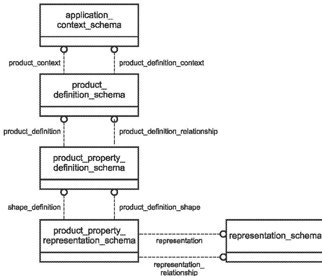
Рисунок D.1 — Структура обобщенного ресурса описания изделия
