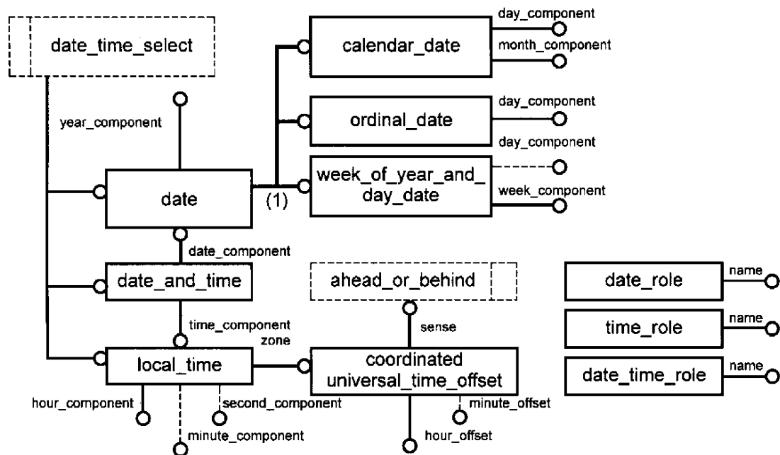
Рисунок F.13 — date_time_schema — EXPRESS-G диаграмма 1 из 1
