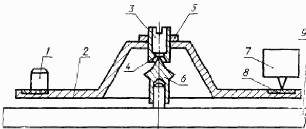
1 — протинавес; 2 — диск; 3 — втулка; 4 — подпятник; 5 — стопорная гайка; 6 — споре; 7 — головка звукоснимателя; 8 — кольцо из материала грампластины; 9 — диск ЭПУ
