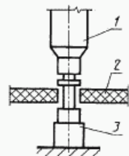
1 — машина; 2 — пол; 3 — нагрузочное устройство
