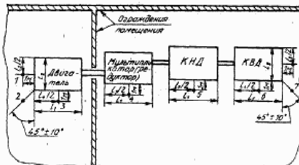
1—7 — точки измерения шума; КНД — корпус низкого давления компрессора; КВД — корпус высокого давления компрессора; L_1 и L_2 — длина и ширина огибающего источника шума параллелепипеда
