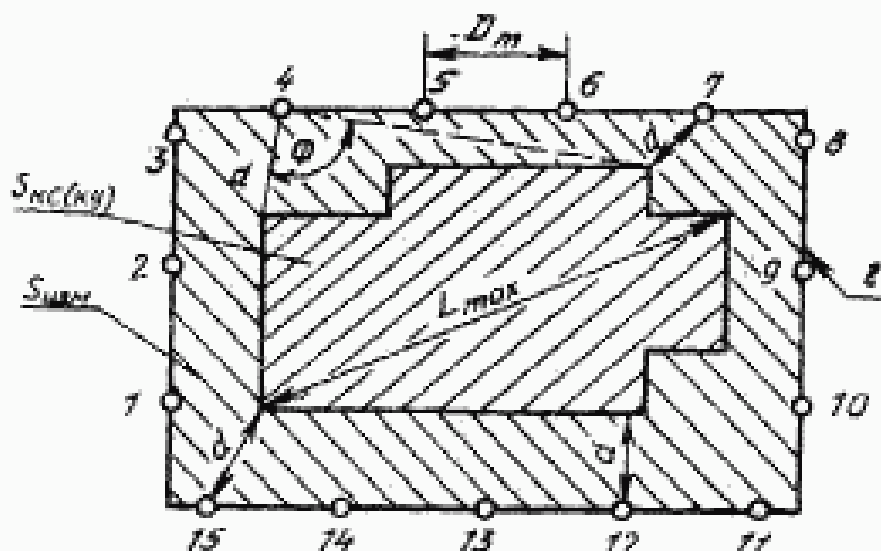
1—16 — точки измерения; \Phi — угол обзора; D_{изм} — расстояние между точками измерения; d — измерительное расстояние; L_{шаг} — наибольший размер по площади КС (КУ); S_{КС(КУ)} — площадь КС (КУ); S_{изм} — измерительная площадь; l — длина измерительного контура
