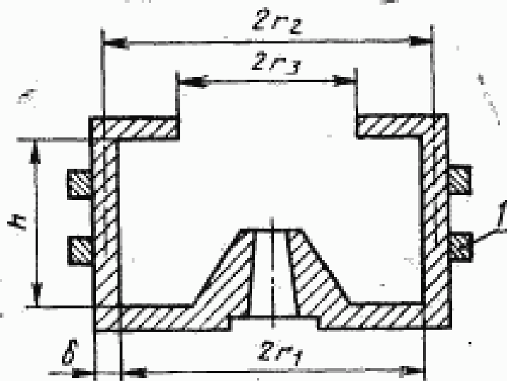
I — поперечное сечение подкрепляющих колец
