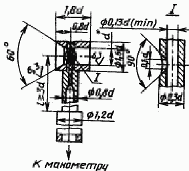
Основные размеры приемной части приемника полного давления
