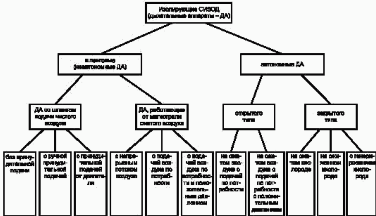
Рисунок 4 — Классификация изолирующих средств индивидуальной защиты органов дыхания
