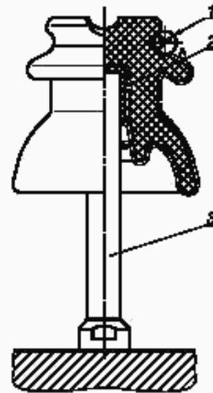
1 — провод; 2 — уплотнитель; 3 — штырь
