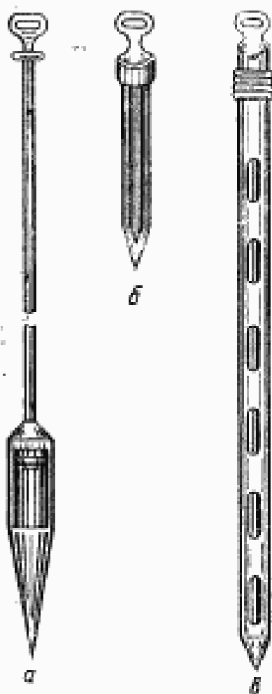
Щупы: а—конусный; б—мешочный; в—цилиндрический
