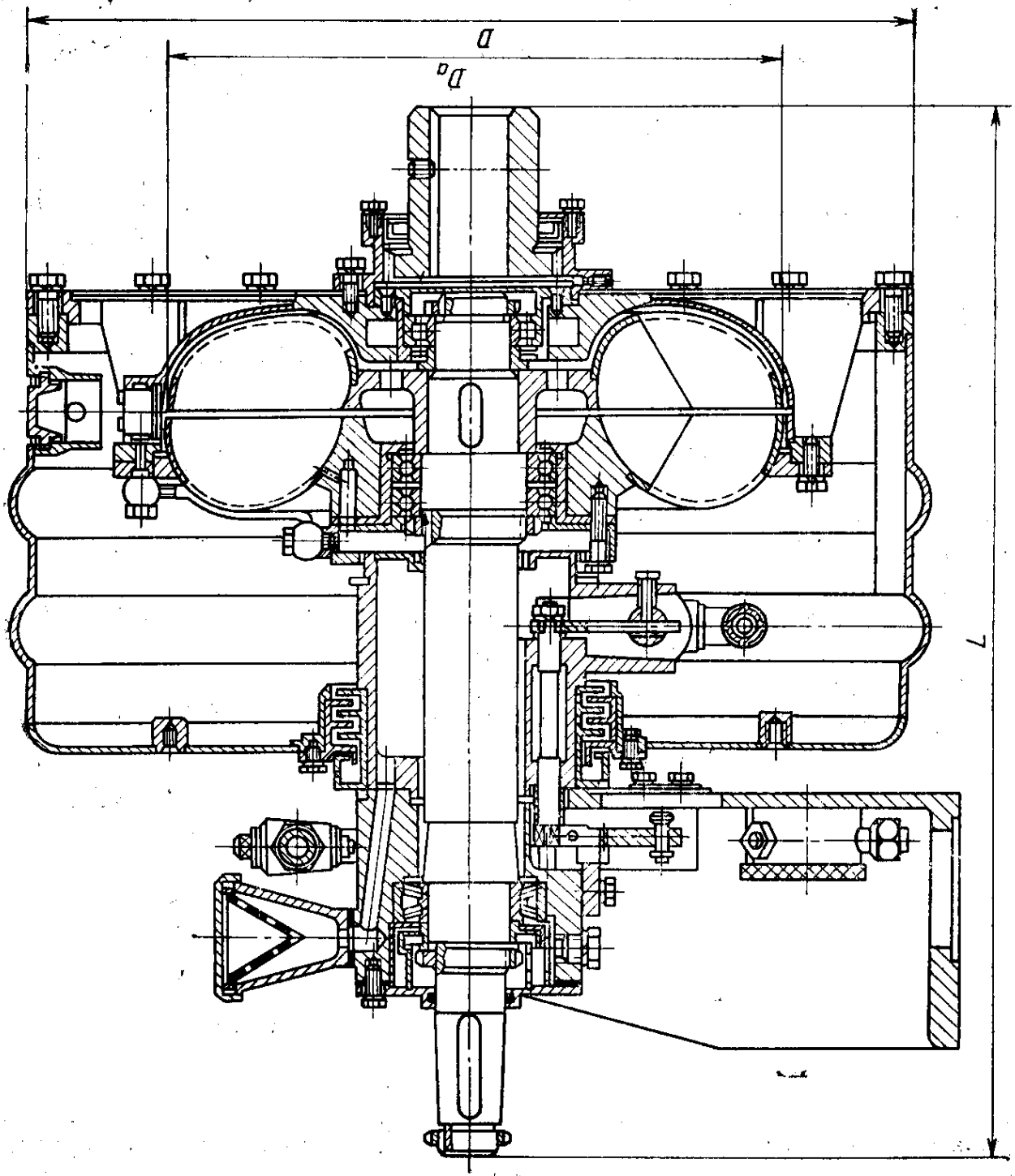
Примечание. Чертеж не определяет конструкцию гидродинамической муфты.
