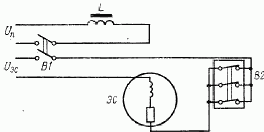
Схема измерения собственного времени отключения
