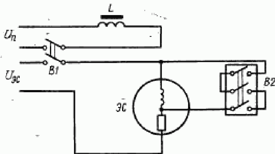
Схема измерения собственного времени включения
