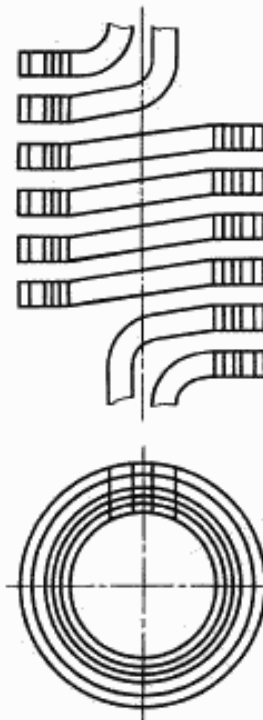
Двухходовая винтовая обмотка трансформатора (к термину 7.2.13)
