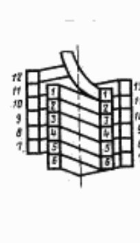
Двухслойная цилиндрическая обмотка трансформатора (к термину 7.2.5)
