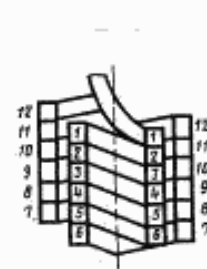
Двухслойная цилиндрическая обмотка трансформатора (к термину 7.2.5)
