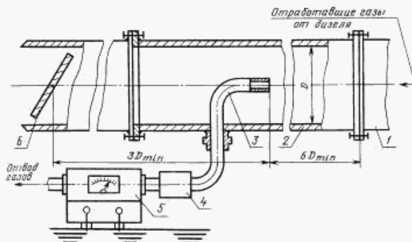
Схема измерения дымности отработавших газов
