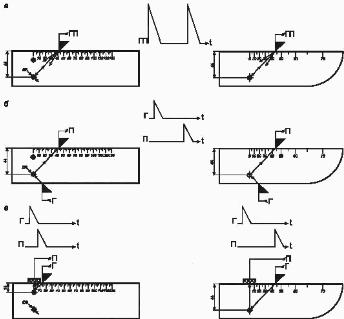
Рисунок 5 — Схема расположения преобразователей на стандартном образце СО-2Р (СО-3Р) при измерении (настройке) условной чувствительности при контроле: a — эхо-методом, b — зеркальным методом, в — дельта-методом
