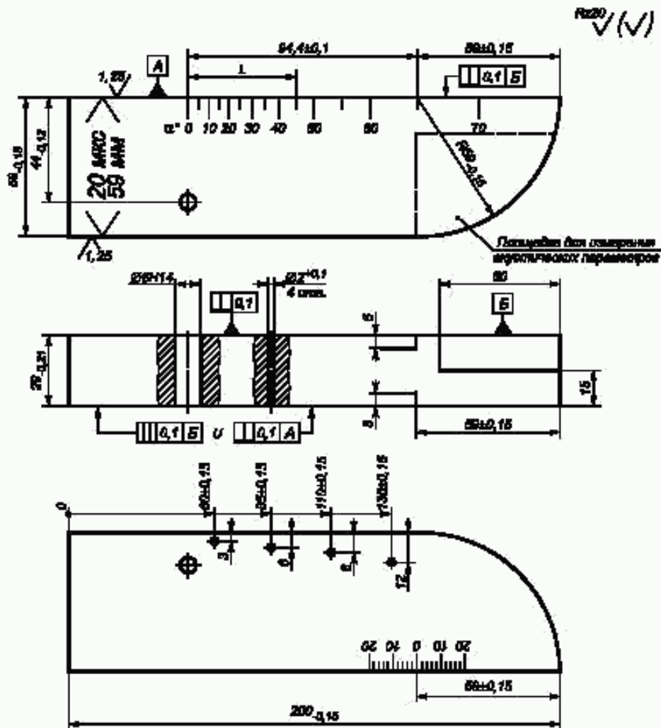
Рисунок 4 — Стандартный образец СО-3Р
