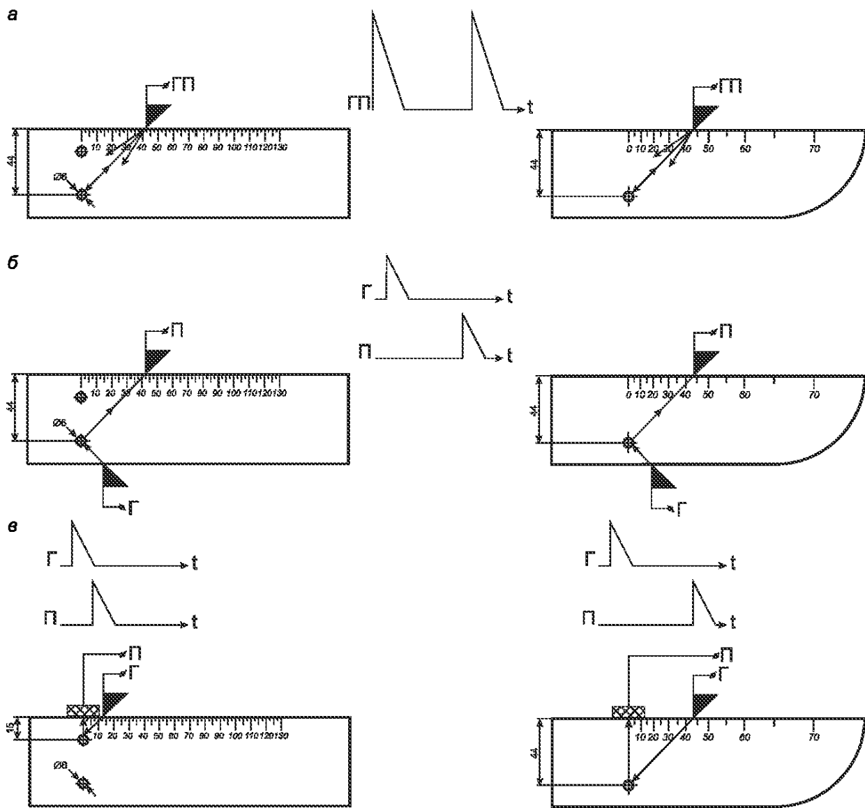
Рисунок 5 — Схема расположения преобразователей на стандартном образце СО-2Р (СО-3Р) при измерении (настройке) условной чувствительности при контроле: а — эхо-методом, б — зеркальным методом, в — дельта-методом
