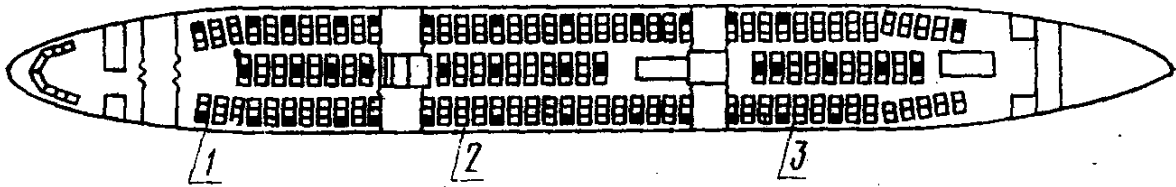
1, 3—салоны туристского класса; 2—салон туристского и экономического классов
