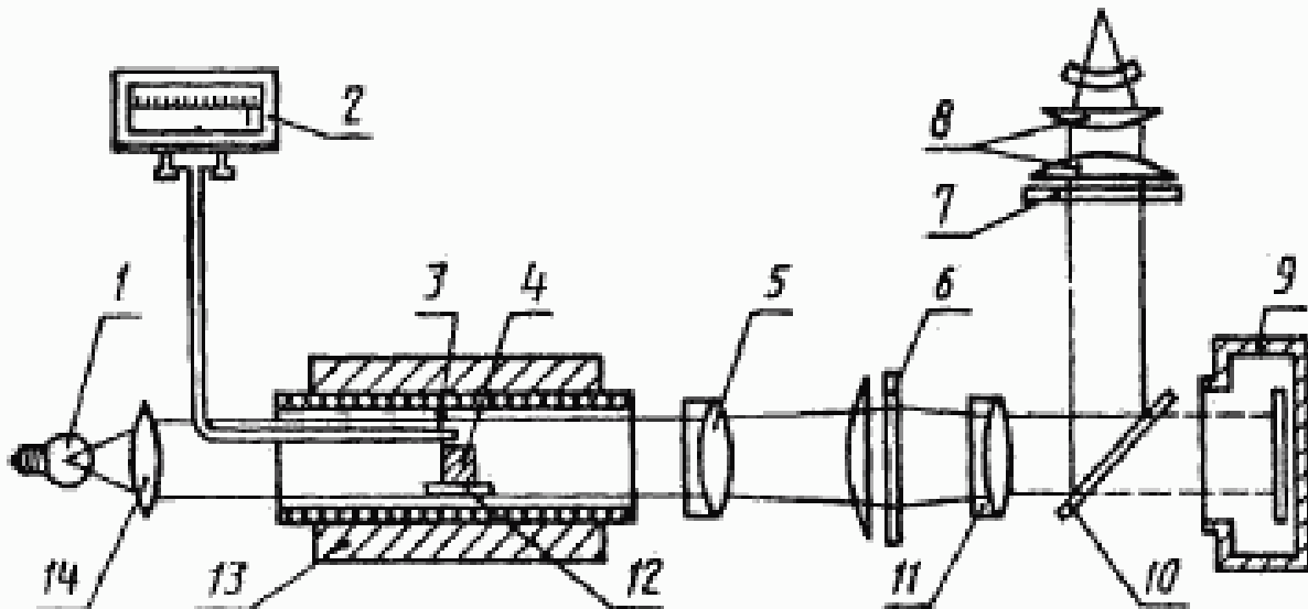
1 — осветитель; 2 — микролинейка; 3 — термометр; 4 — образец из золы; 5 — координатная сетка; 6 — выпуклая линза; 7 — корпус микроскопа; 8 — объектив микроскопа; 9 — фотоаппарат; 10 — призма; 11 — выпуклая линза; 12 — подставка; 13 — основание микроскопа; 14 — конденсор
