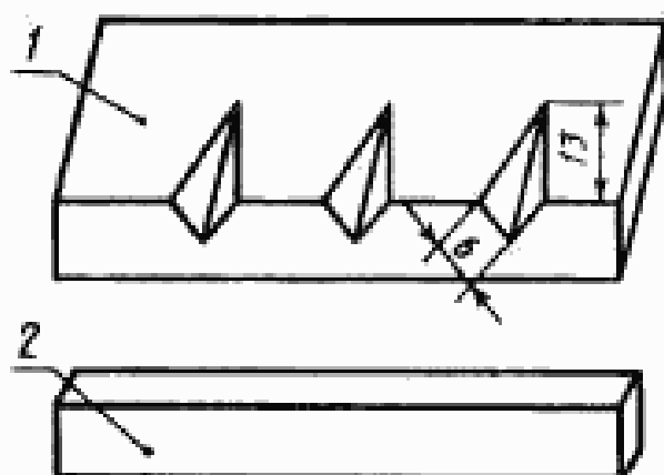
1 — форма для изготовления образцов золы; 2 — крышка (формулы) пластинки к форме
