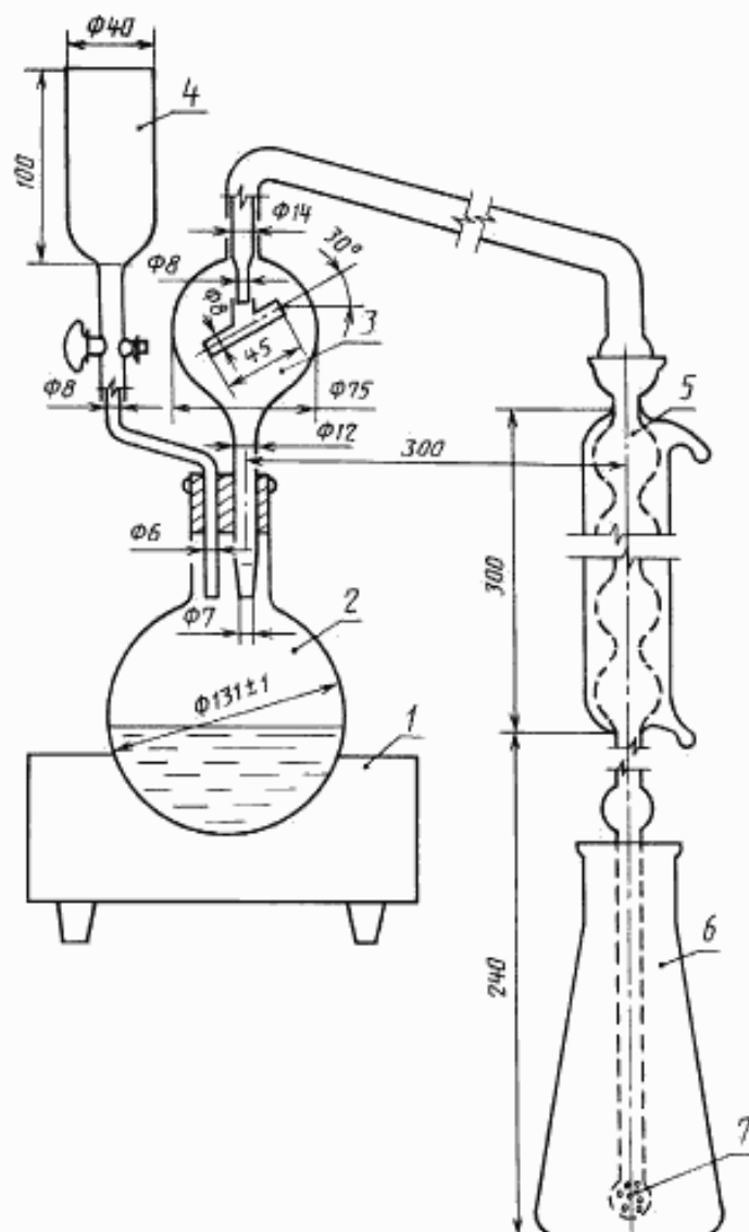
1 — колбонагреватель; 2 — реакционная колба вместимостью 0,5—1,0 дм 3 ; 3 — каплеуловитель; 4 — капельная воронка с краном; 5 — холодильник; 6 — приемник; 7 — барботер
