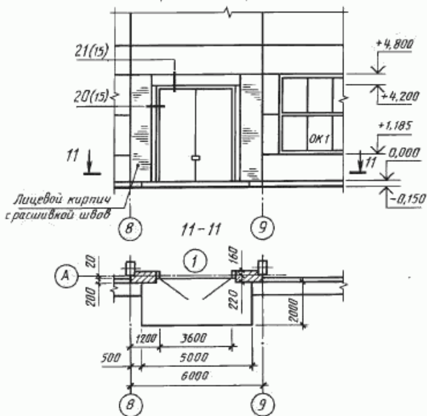
Фрагмент 3 фасада
