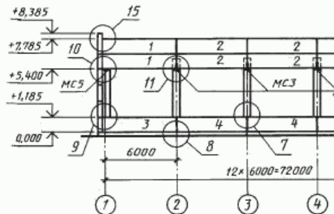
Схема расположения панелей стен
