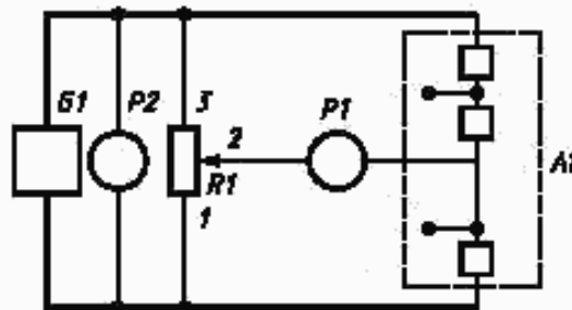
G1 — источник напряжения постоянного тока; R1 — проверяемый резистор; P1 , P2 — вольтметр постоянного тока; A1 — образцовый делитель напряжения или другое устройство, формирующее образцовую функциональную характеристику
