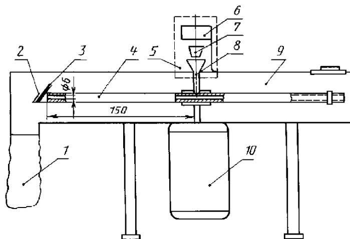
Рисунок 1 — Центробежный абразивметр
