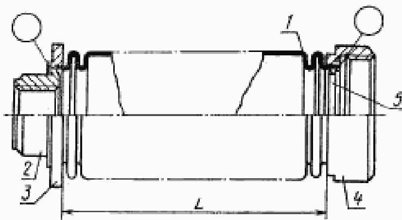
1—сильфон; 2—штулка; 3—кольцо; 4—штулка; 5—кольцо
