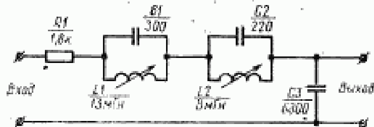
Электрическая схема фильтра нижних частот
