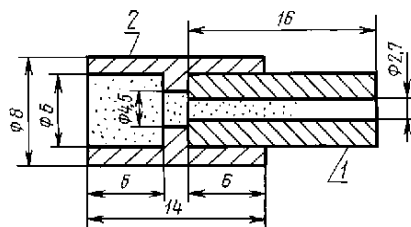
1 — нижняя часть электрода, зажимаемая в электрододержателе; 2 — насадка
