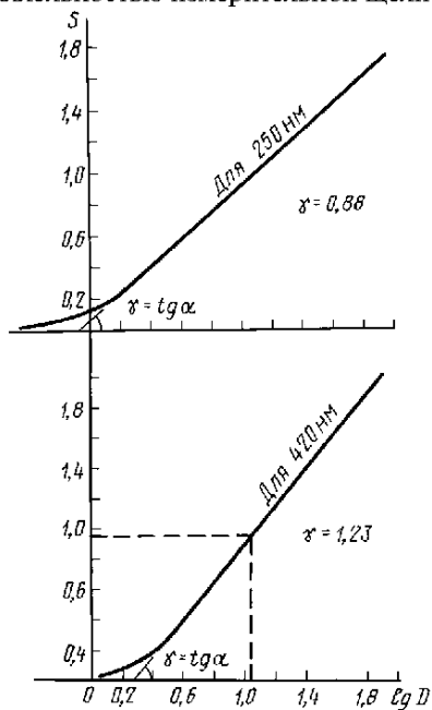
Характеристические кривые фотопластинок типа «Микро»
