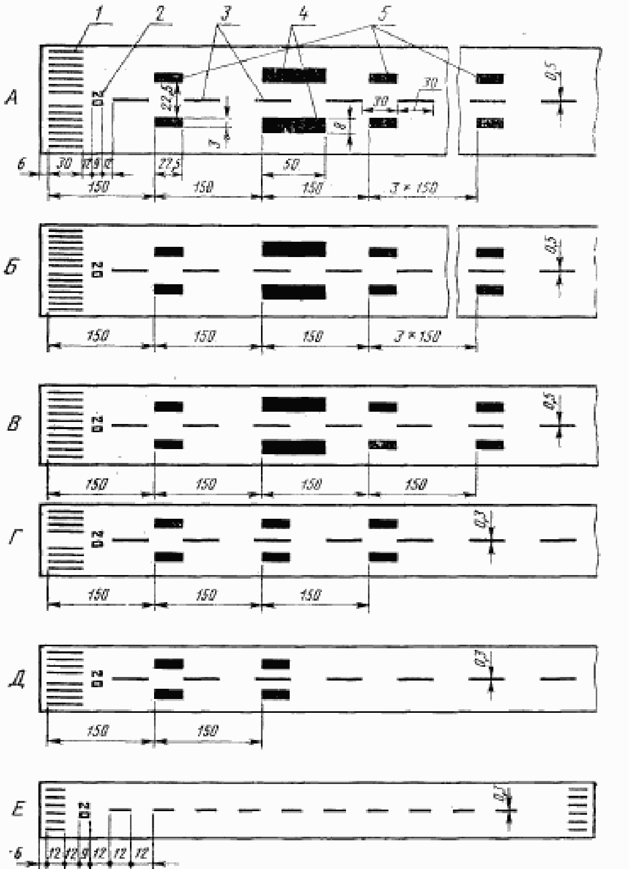
А, Б, В, Г, Д и Е — варианты аэродромов: 1 — ворота; 2 — цифровой знак ПМПУ; 3 — ось ИВПП; 4 — фиксированное расстояние; 5 — зона приземления
