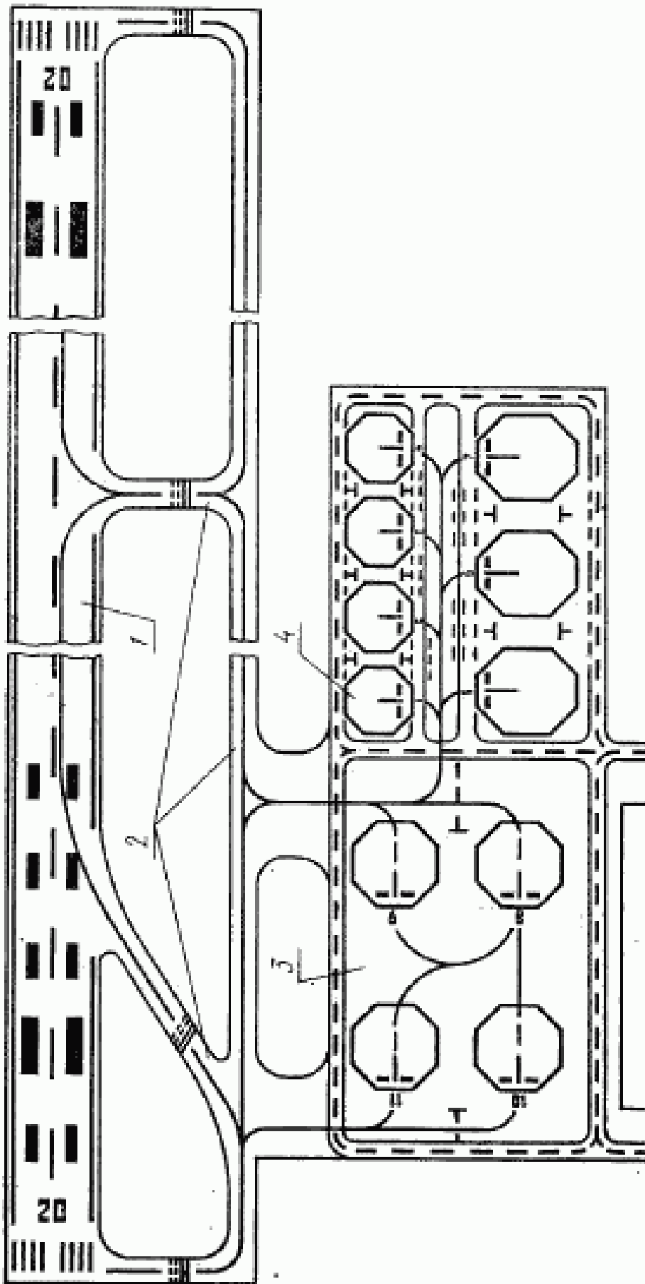
1—искусственная волново-ребристая полоса; 2—рулежные дорожки; 3—вертол; 4—места стоянки Черт. 1
