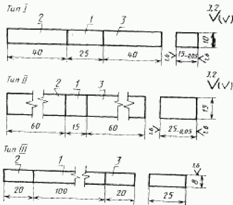
Заготовки составных образцов для наплавки валика
