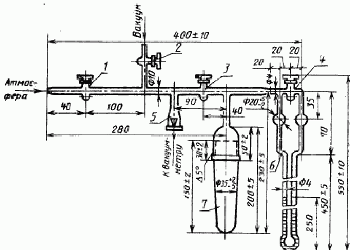
1, 2, 3, 4 — краны вакуумные; 5 — лампа вакуумметрическая; 6 — манометр; 7 — колба
