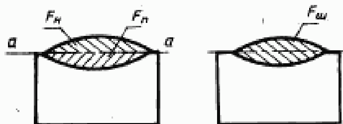
Поперечное сечение образца
