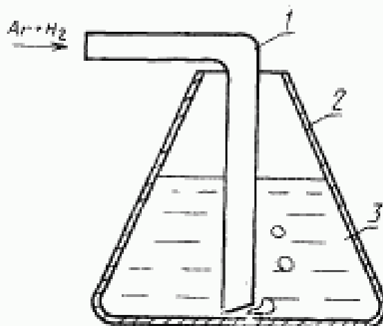
Схема устройства для набора ПГС в шприц
