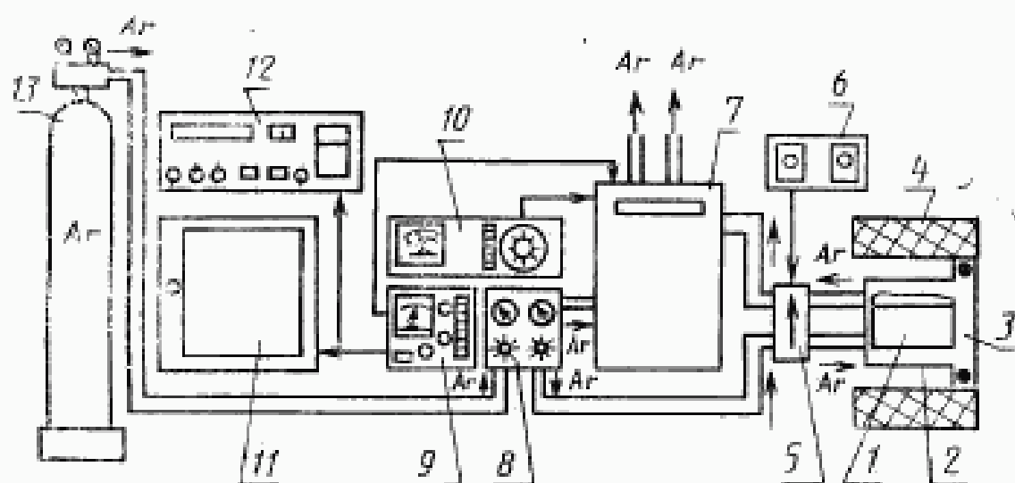
Схема прибора для хроматографического метода анализа (метод 1)
