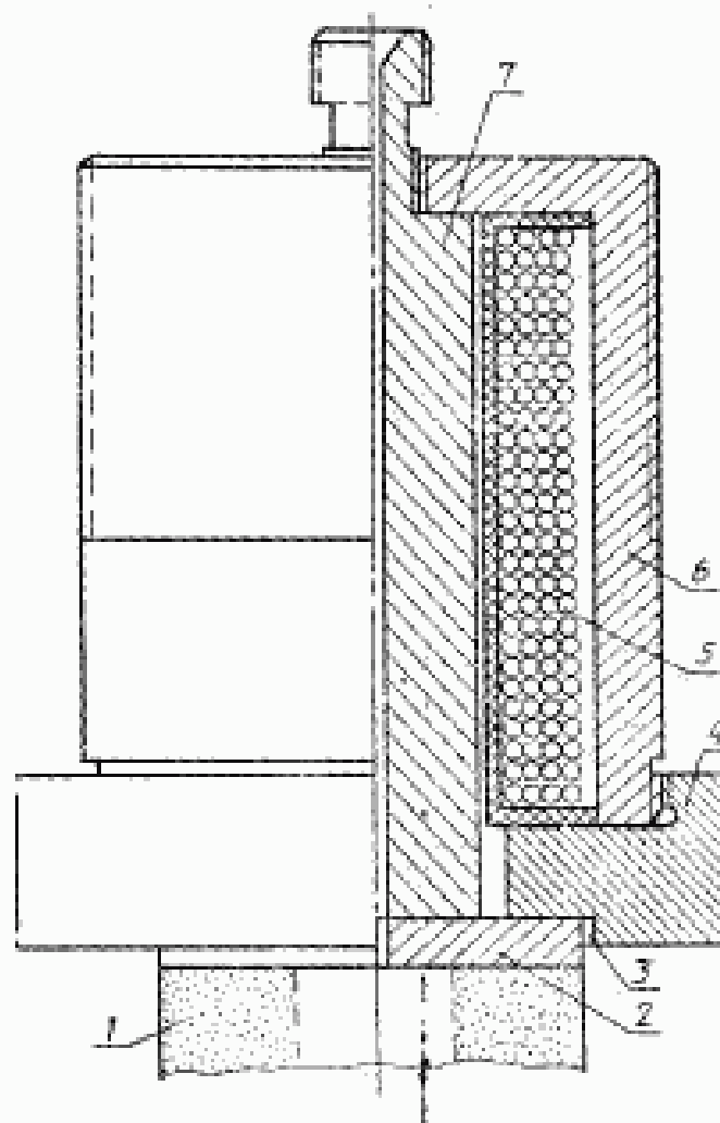
Схема магнитного захвата
