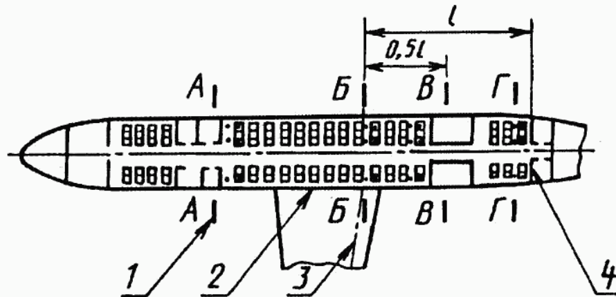
A, B, B, Gamma — сечения; 1 — плоскость вращения внутренних винтов; 2 — корневая нервюра; 3 — задний лонжерон; 4 — задняя стенка пассажирской кабины Черт. 5
