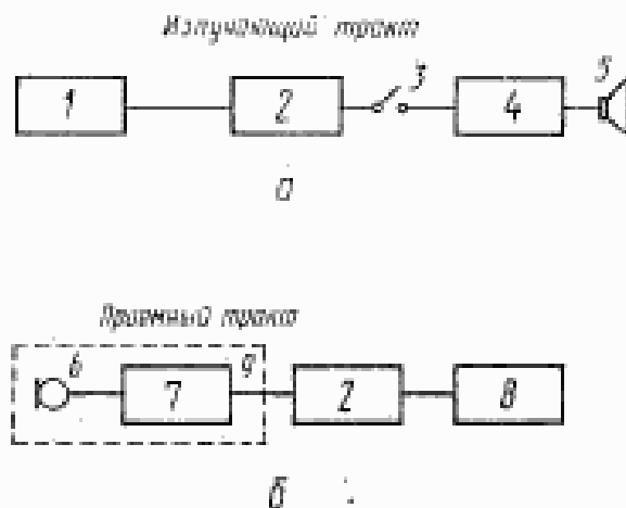
Блок-схема аппаратуры для измерения времени реверберации
