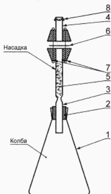
1 — коническая колба с плоским дном; 2 — резиновая пробка; 3 — длинная трубка; 4 — короткая трубка; 5 — вата; 6 — бумажный фильтр; 7 — резиновые кольца; 8 — бумажный колпачок
