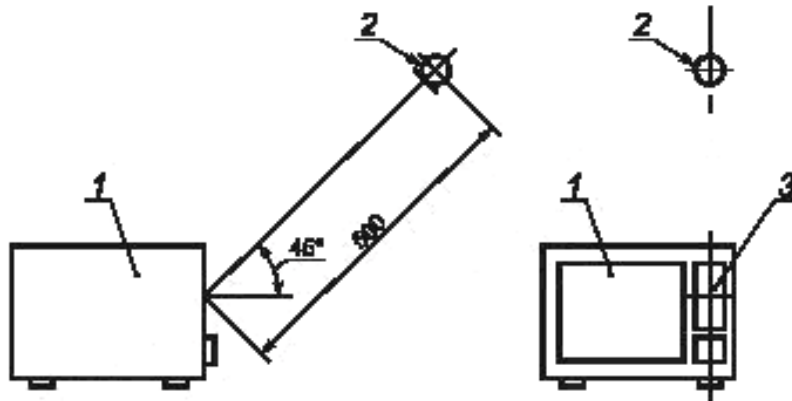
а) Блок управления параллельно расположен на лицевой стороне изделия: оправа — вид сбоку, оправа — вид спереди
