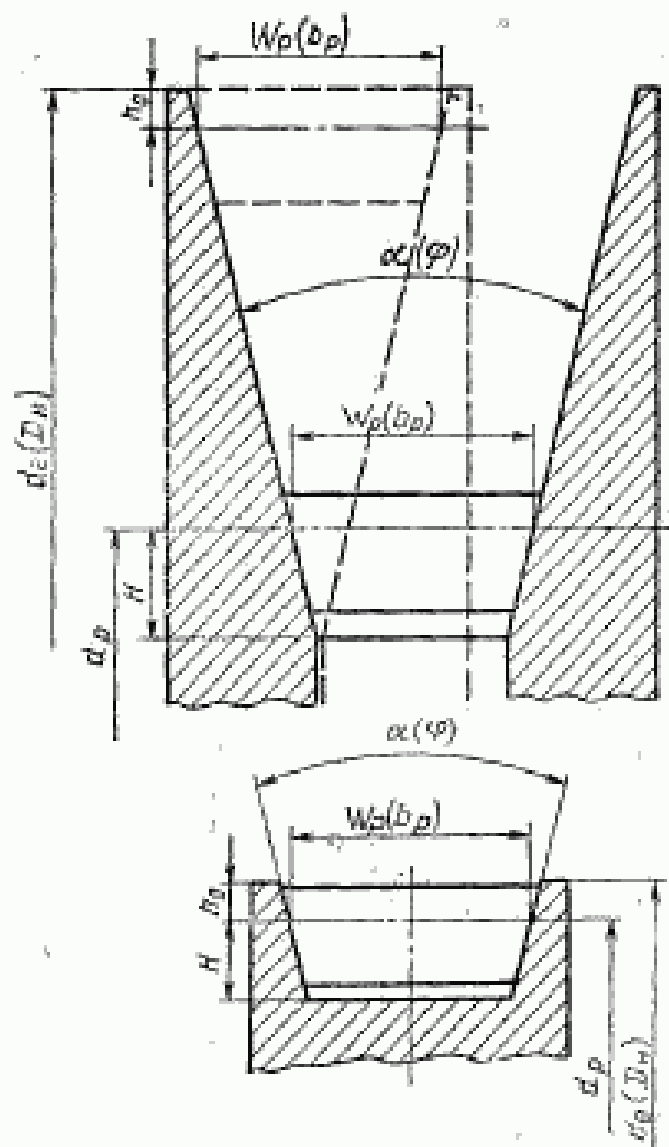
d_e(D_n) — наружный диаметр шкива; d_p — расчетный диаметр шкива
