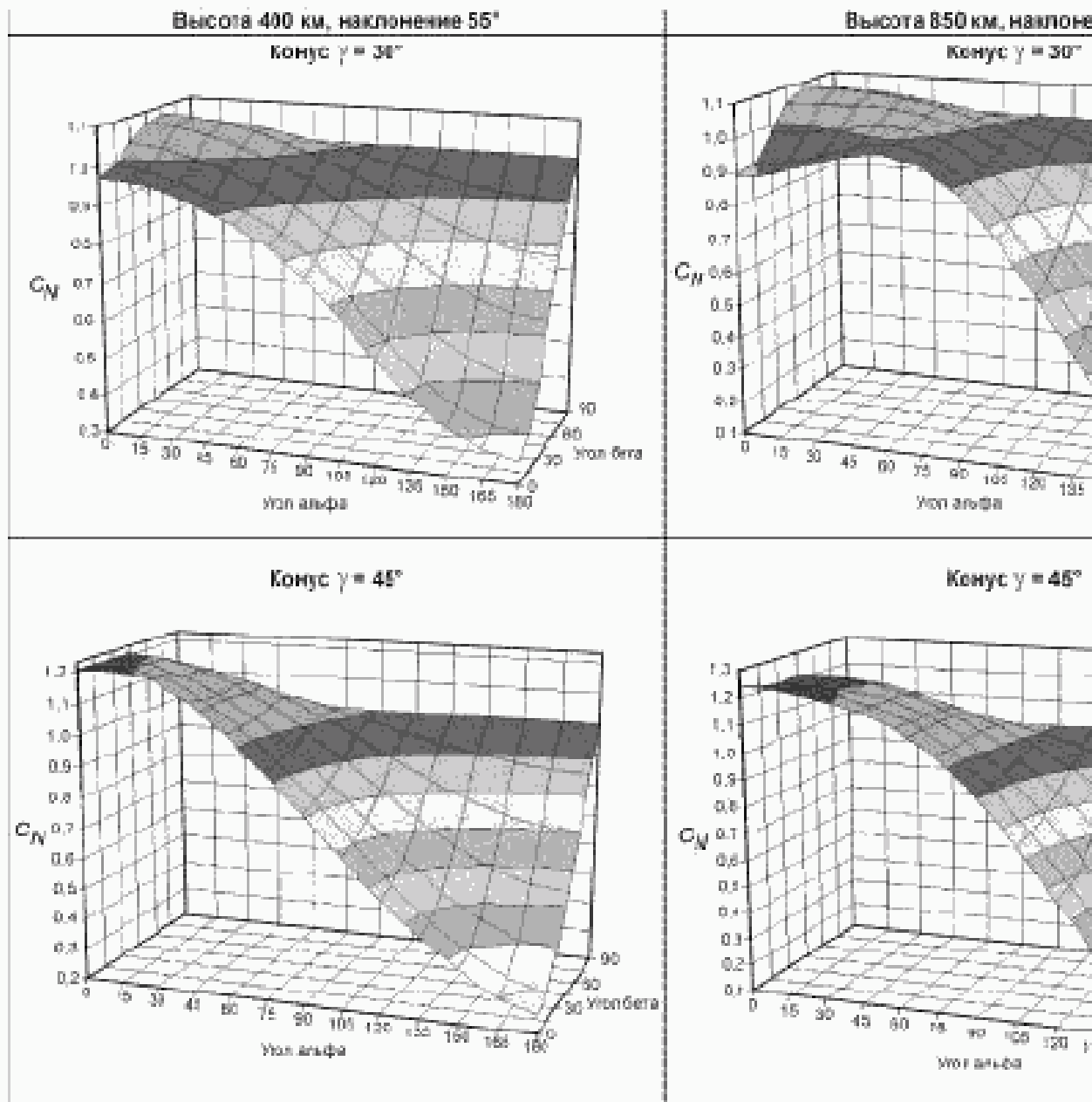
Рисунок 7.4 — Зависимость коэффициента C_N от ориентации
