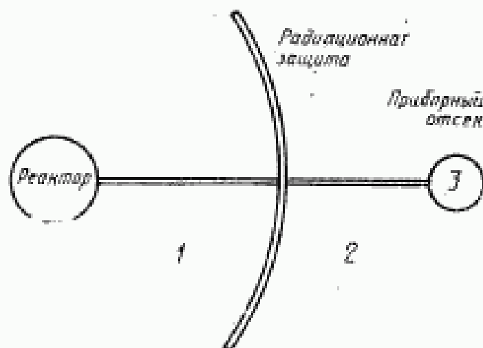
Рисунок 1 — Схема космического аппарата с бортовым ядерным реактором
