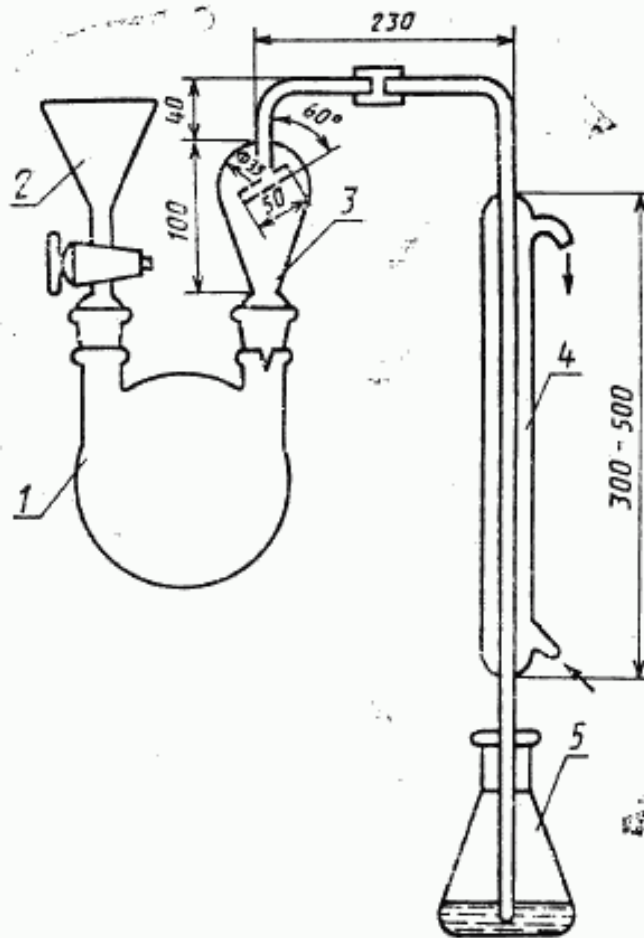
1—двухгорловая колба вместимостью 750 см 3 ; 2—воронка; 3—каплеуловитель; 4—холодильник; 5—приемник вместимостью 500 см 3
