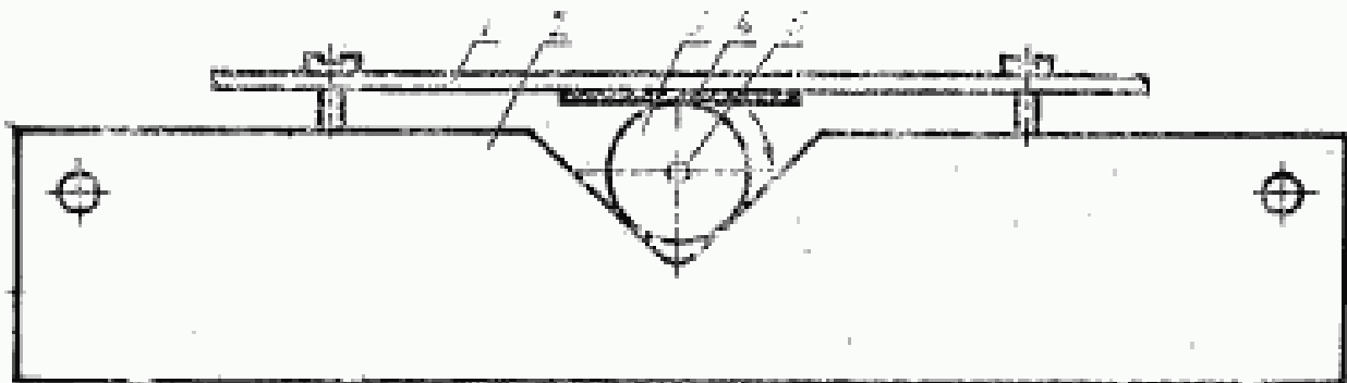
1 — прижки; 2 — призма; 3 — наконечник; 4 — прокладка; 5 — сердцевина волокна
