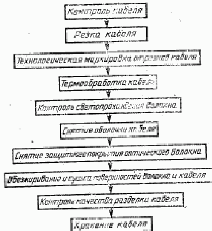
Схема технологического процесса разделки оптического кабеля
